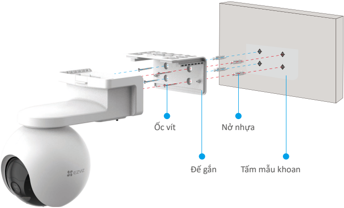
Hình 2 Gắn tường
