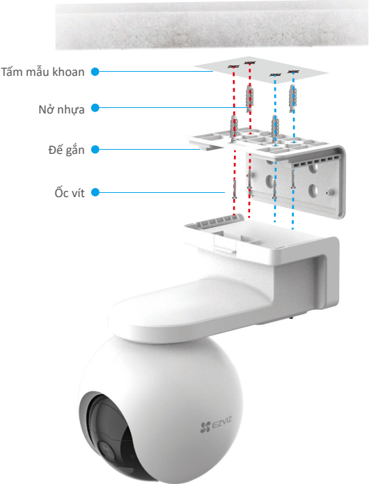
Hình 1 Gắn trần
